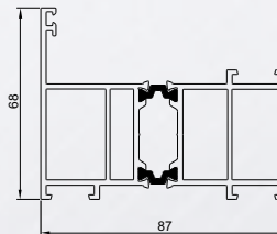
Profil progów ENERGY 90
