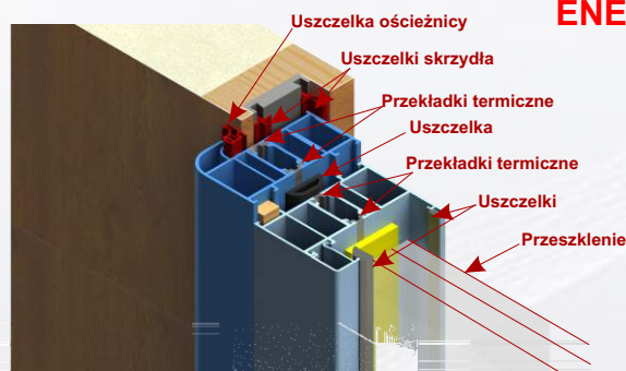
SKRZYDŁO KMT PLUS 75 passive PROFIL OŚCIEŻNICY ENERGY 90 + PROFIL NAŚWIELTA
