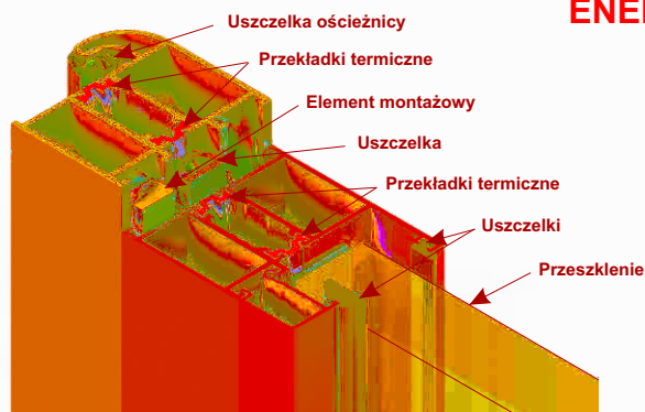
PROFIL OŚCIEŻNICY ENERGY 60 PROFIL NAŚWIELTA
