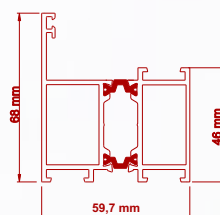
Profil progów ENERGY 60
