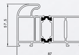
Profil ościeżnicy KMT ENERGY 90
