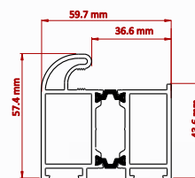
Profil ościeżnicy KMT ENERGY 60
